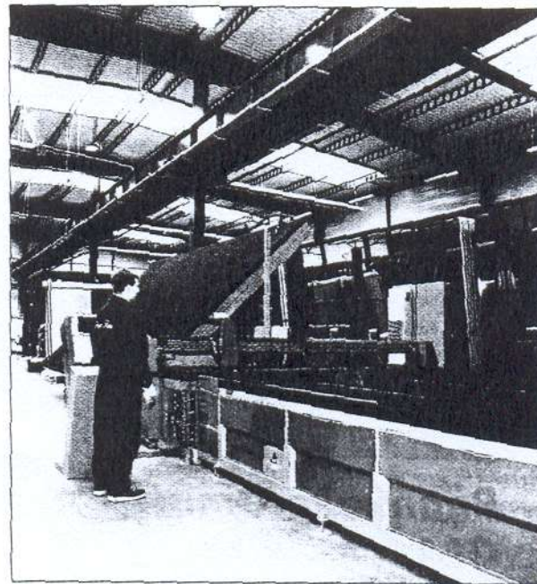
Stół do cięcia laminatów z tafli jumbo
